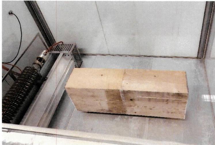
Abbildung 1: Die Probe 1414/2021 in der 1m 3 Prüfkammer
