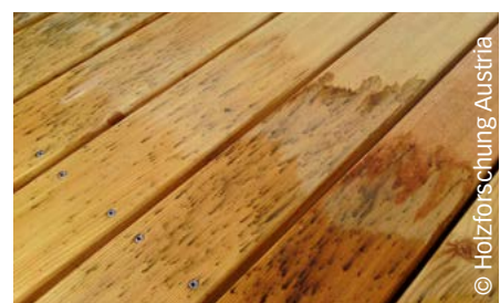
Wasserlösliche Gerbstoffe reagieren bereits beim Kontakt mit minimalen Eisenkonzentrationen. Diese Reaktionen führen zu graublauen bis schwarzen Verfärbungen.
